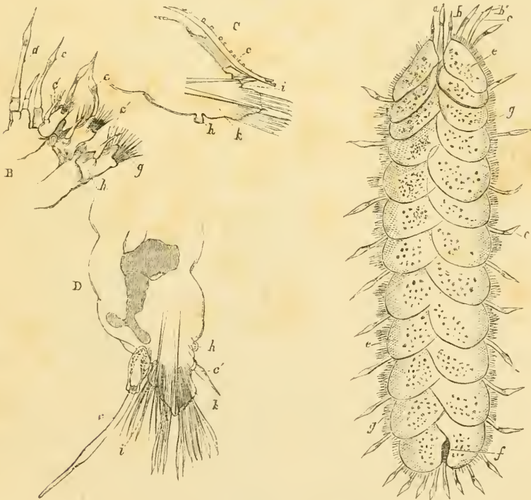
Fig. 24.— Polynöe squamata .
