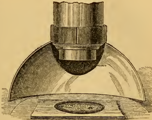
Beck's Parabolic Speculum.
