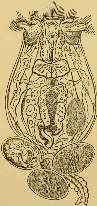
Brachionus pala.
