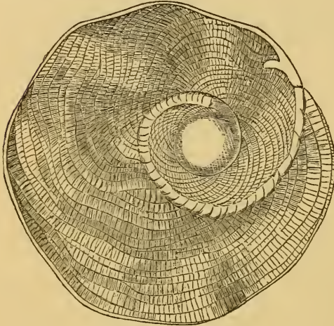
Heterostegina.
