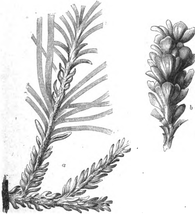
Fig. 59. Voltzia heterophylla .
