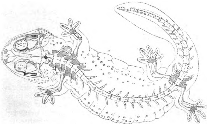
Fig. 72. Andrias Scheuchzeri.
