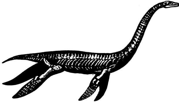
Fig. 66. Plesiosaurus dolichodeirus .
