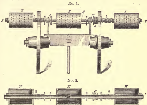
FIG. 58.—N. A. Davis' sifter.
