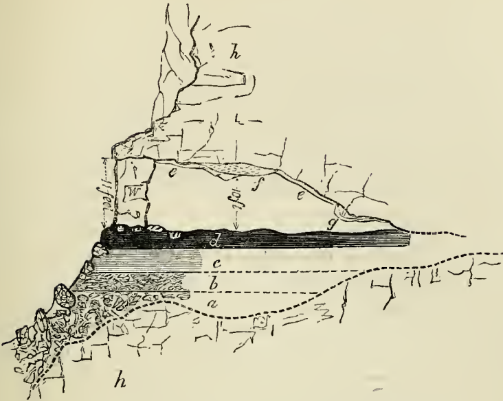
VERTICAL SECTION OF THE GROTTA DI MACCAGNONE.
