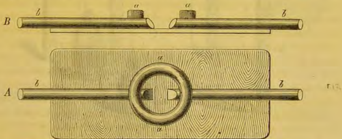
Fig. 1. Gaskammer in natürlicher Grösse. A Vogelperspective. B Mittlerer Längsschnitt. aa Wall. bb Zuleitungsröhren.
