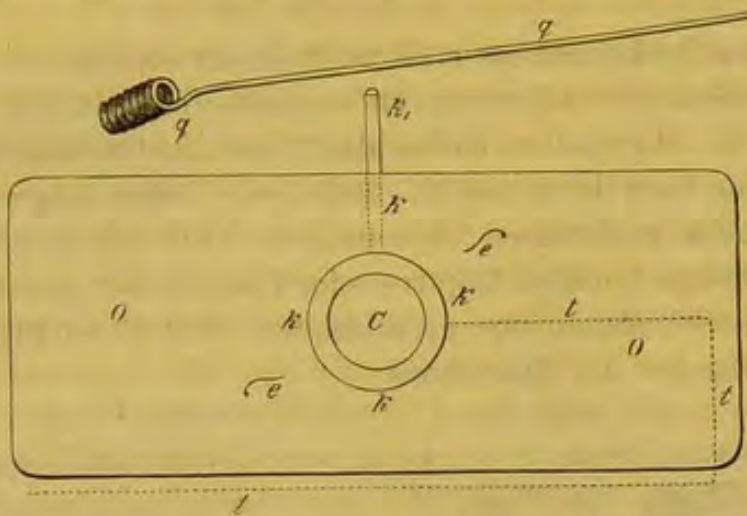
Fig. VII. Heizbarer Objectträger, nat. Grösse. kkkk Kupfer-ring und Streifen in der Platte oo eingeschliffen. q Heizstab. ee Klemmen.
