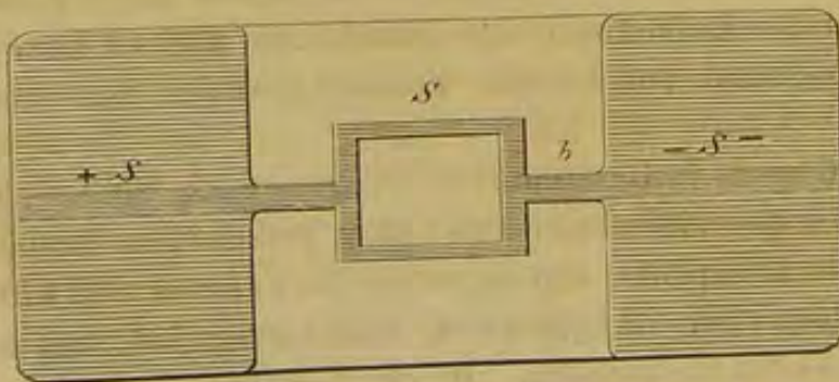
Fig. IV. Objectträger zur elektrischen Heizung, natürliche Grösse.
