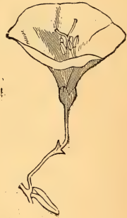
FIG. 243.—Infundibuliform corolla of Convolvulus arvensis .
