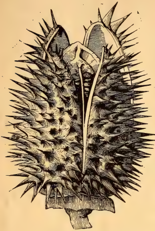
FIG. 310.—Septifragal capsule of Datura .
