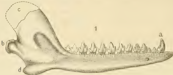
Fig. 1. Rechte Unterkinnlade von Diplocynodon victor Marsh. Äußere Ansicht. (2/1.) a Eckzahn, b Kondylus, c Kronenfortsatz, d Untertieferwinkel.
