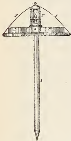
FIG. 79.—THE GARRETT LAMP.
